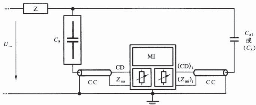
图 1c 平衡试验回路
