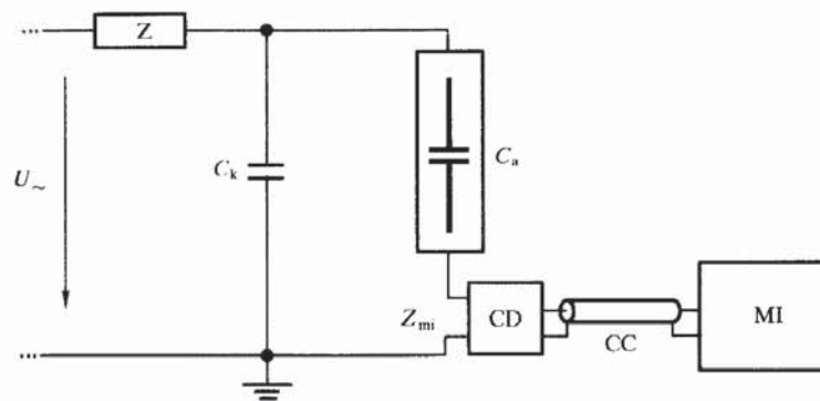
图 1b 耦合装置 CD 与试品串联
