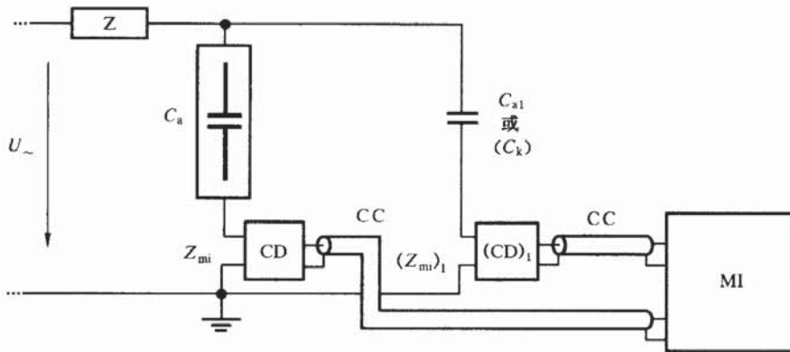
图 1d 极性辨别回路
